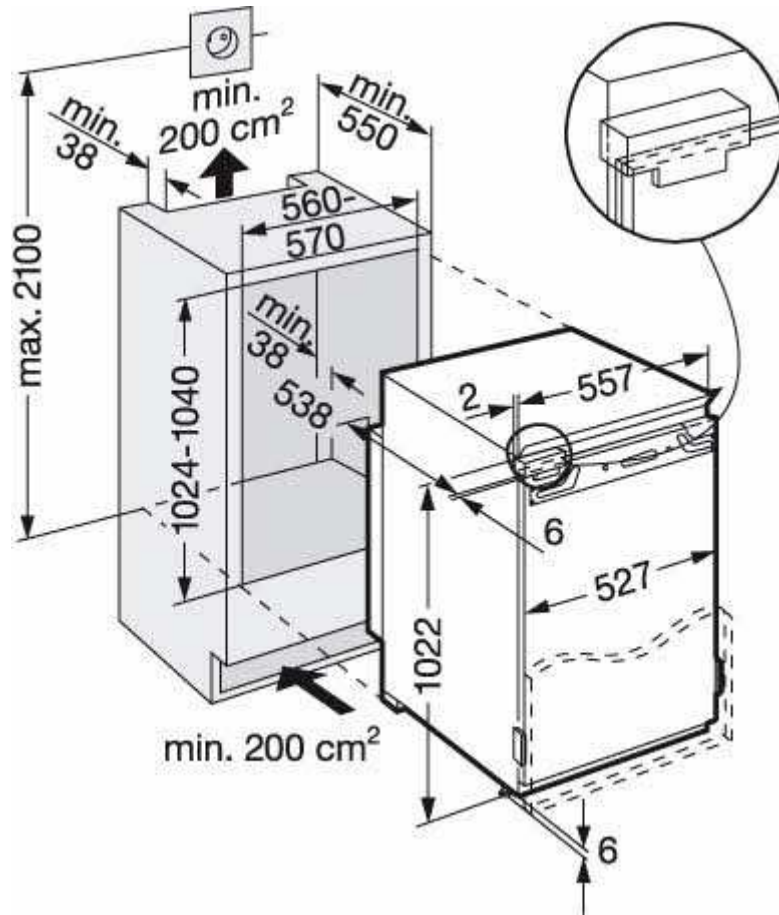
Einbauskitze
